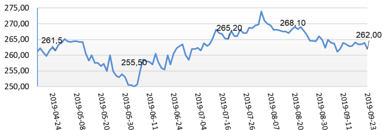
RTT - kontrakt BASE I kw. - 2020 (PLN/MWh)
